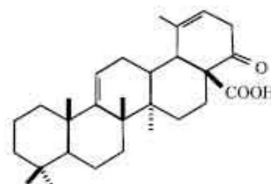
FIG. 3: BRYOPHOLLONE
