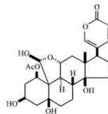
FIG. 1: BRYOPHYLLIN
