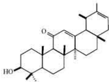
FIG. 5: BRYOPHYNOL
