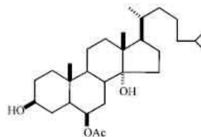
FIG. 2: BRYOPHYLLOL
