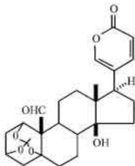
FIG. 6: BERSALDEGENIN
