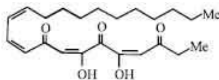
FIG. 4: BRYOPHOLLENONE
